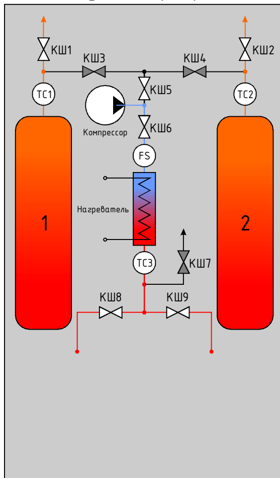
Режим регенерации двух адсорберов
